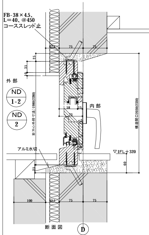
ND-1・2 テラス戸 縦断面図
