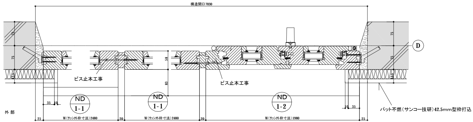
ND-1 横断面図
