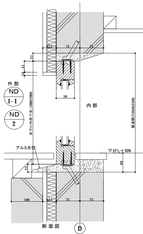
ND-1・2 FIX 縦断面図
